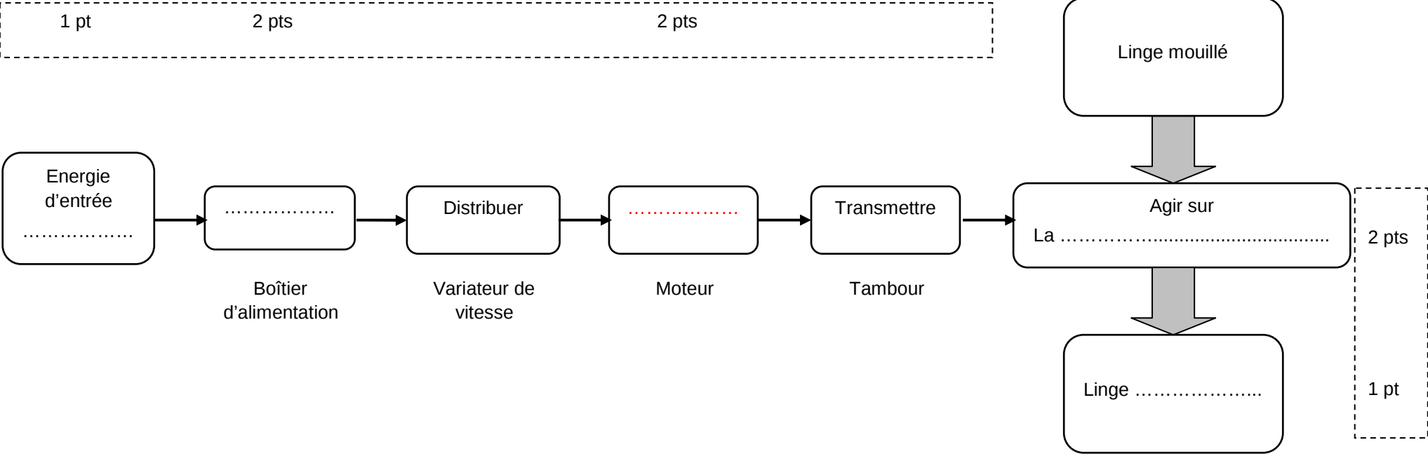
Document 3 : Chaine d'énergie du lave-linge
