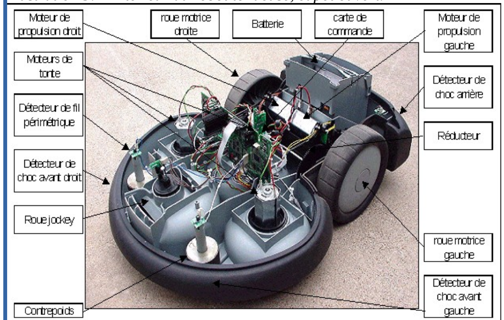
Illustration 3: L'intérieur du robot tondeuse, capot ouvert.
