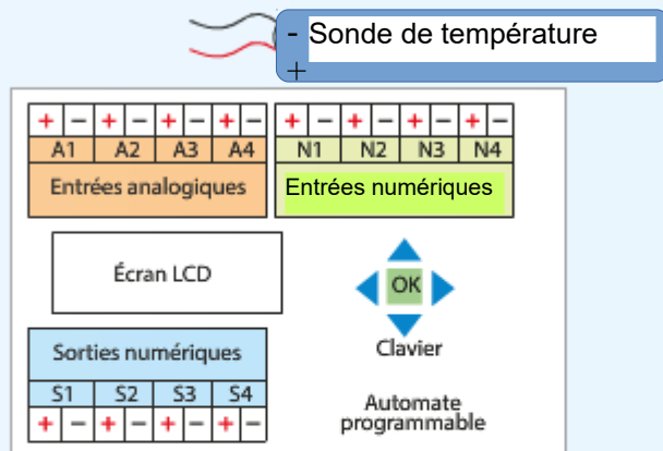
Doc. 3 Plan de câblage du système automatisé
